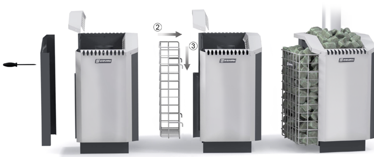
Рисунок - 6. Установка сетки-каменки на печь
