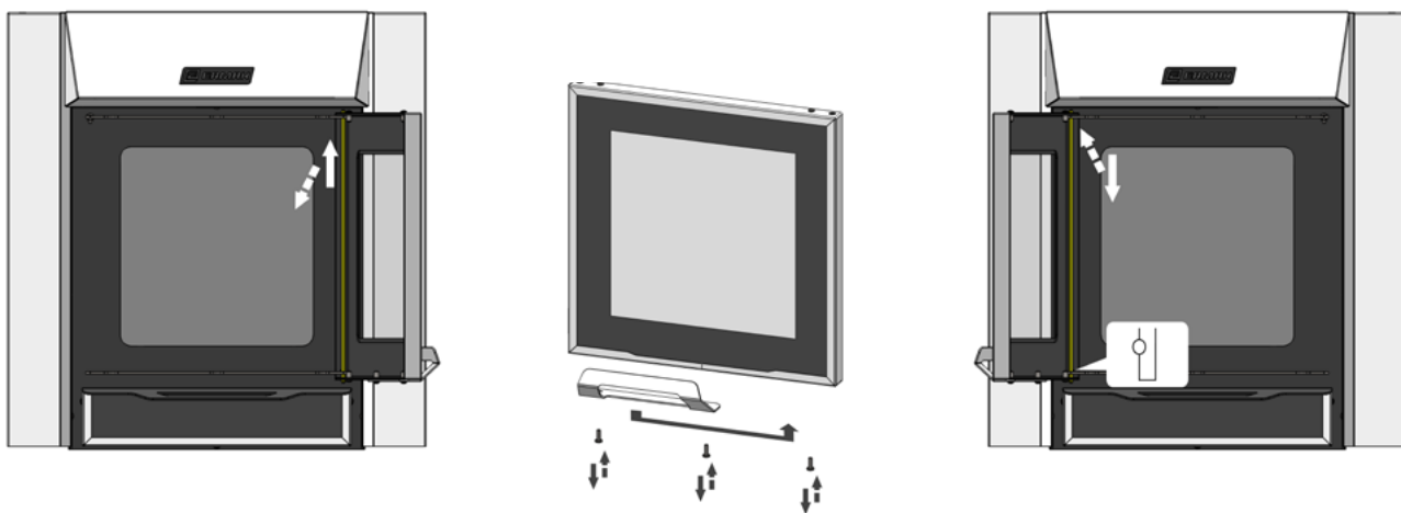
Рисунок - 4. Схема снятия и изменения открытия дверки
